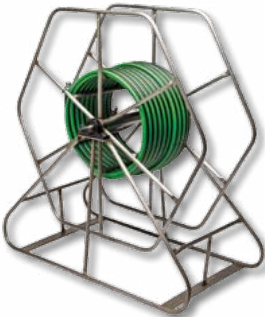
Soporte de carrete de manguera completo con doble línea de descenso para el uso con equipos offshore.
