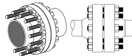
Tensionado de un 50% de los pernos
